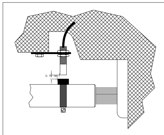
Рис. 5-1 Датчик Х на карданном валу
