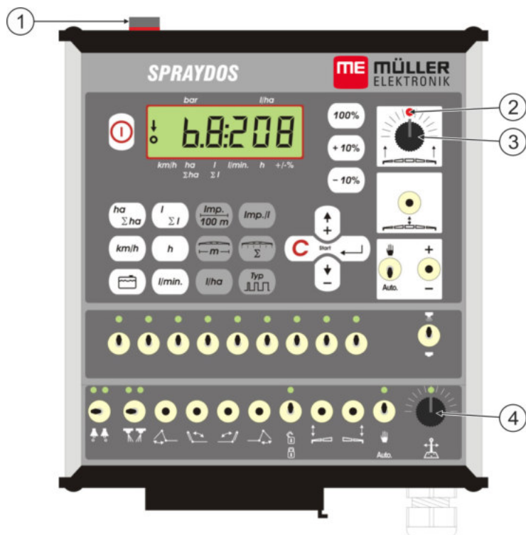
Рис. 6-3 Эксплуатационные элементы, необходимые для калибровки
