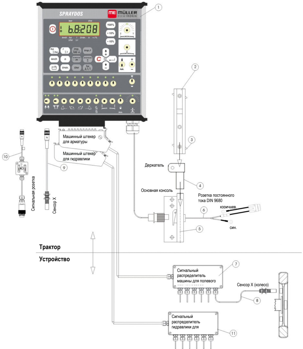
Рис. 4-1 Обзор SPRAYDOS
