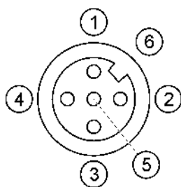
Raspored pinova utičnice (u terminalu)
