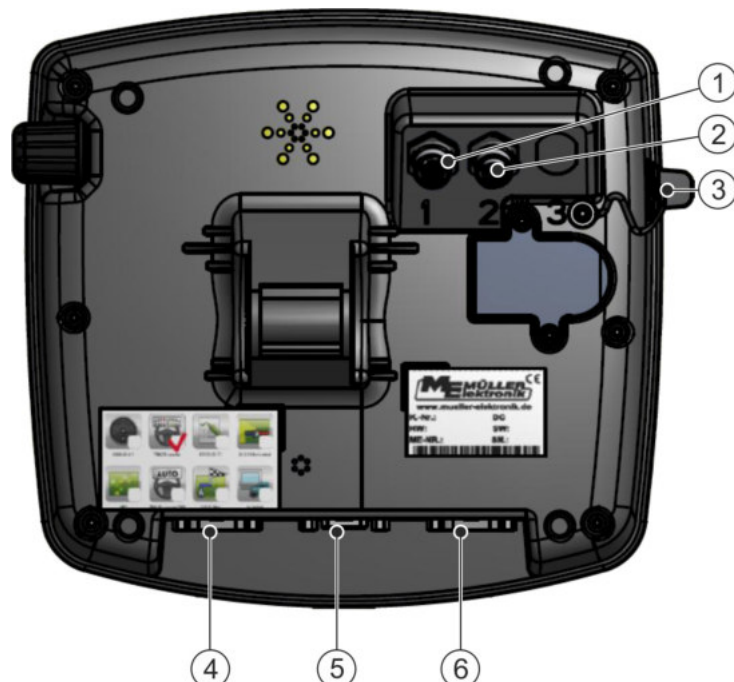
A terminál hátoldala Kameracsatlakozásokkal változat
