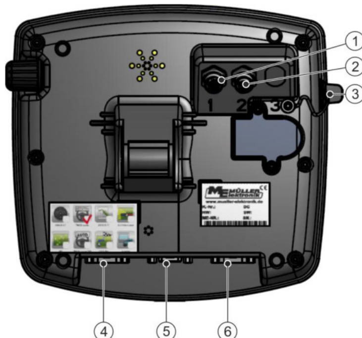
Zadná strana terminálu. Variant s kamerovými konektormi.
