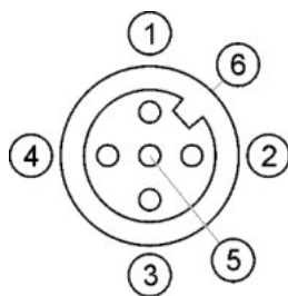
Obsadenie pinov zásuvky (v termináli)
