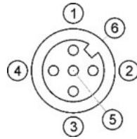
Yuvanın (terminalde) pin ataması
