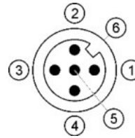
Konnektörün pin ataması
