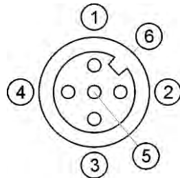
M12-utičnica: Ethernet
