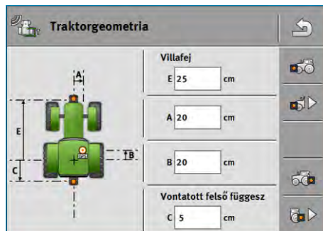
Traktorgeometria (példa)
