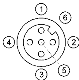
Liidese kontaktide paigutus (terminalis)
