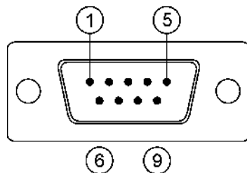
9-klemmine D-Sub-pistik
