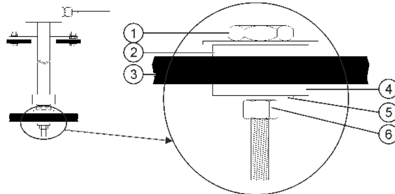
Rohrhalterung montieren
