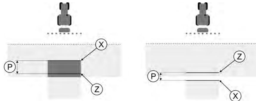
Linien für den Parameter "Trägheit Korrektur bei Aus". Links: Feldspritze schaltet zu spät aus. Rechts: Feldspritze schaltet zu früh aus.
